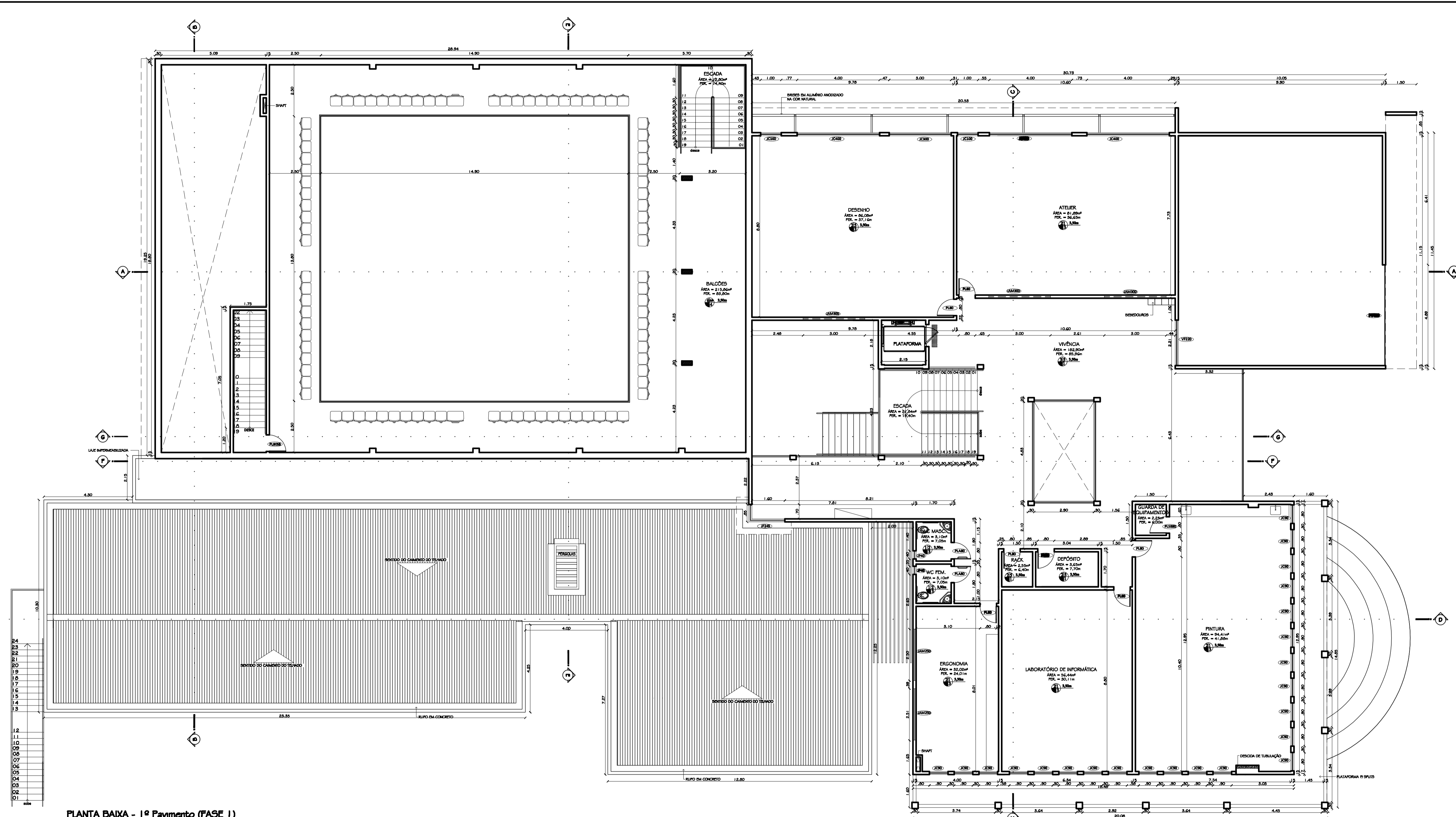
PLANTA BAIXA - 1º Pavimento (FASE I) ESCALA 1/75
